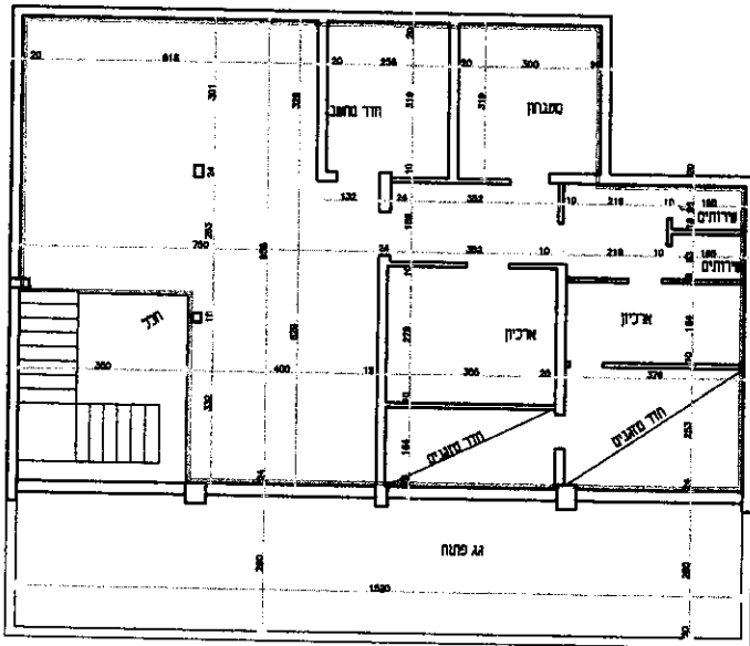
כניית קומה א קנ"מ 1:100
